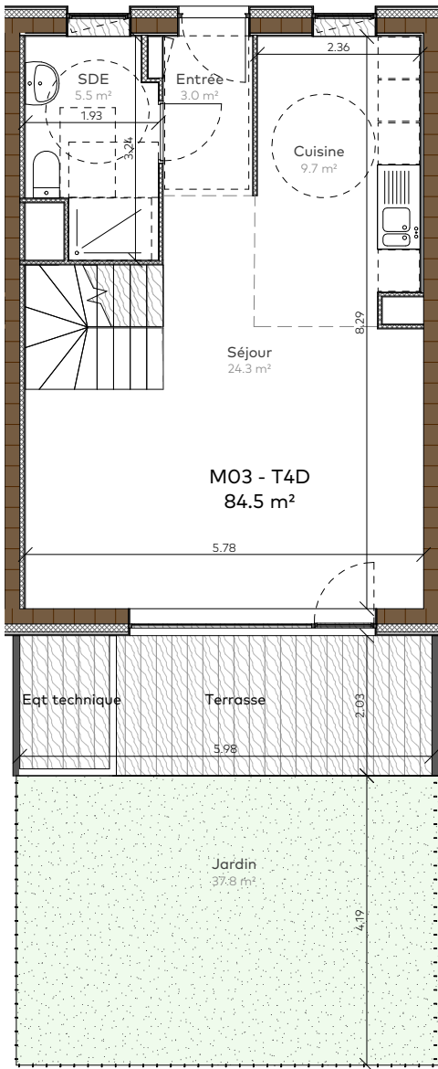
Plan RDC
