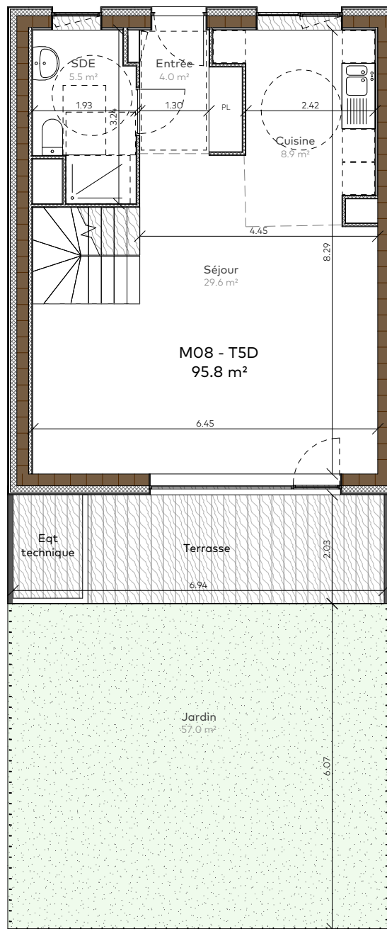
Plan RDC
